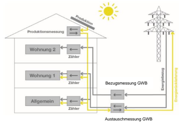
Abbildung 2: Messgeräteanordnung 2
