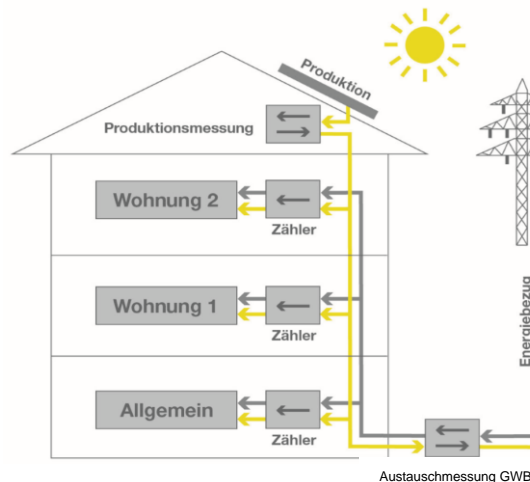
Abbildung 1: Messgeräteanordnung 1
